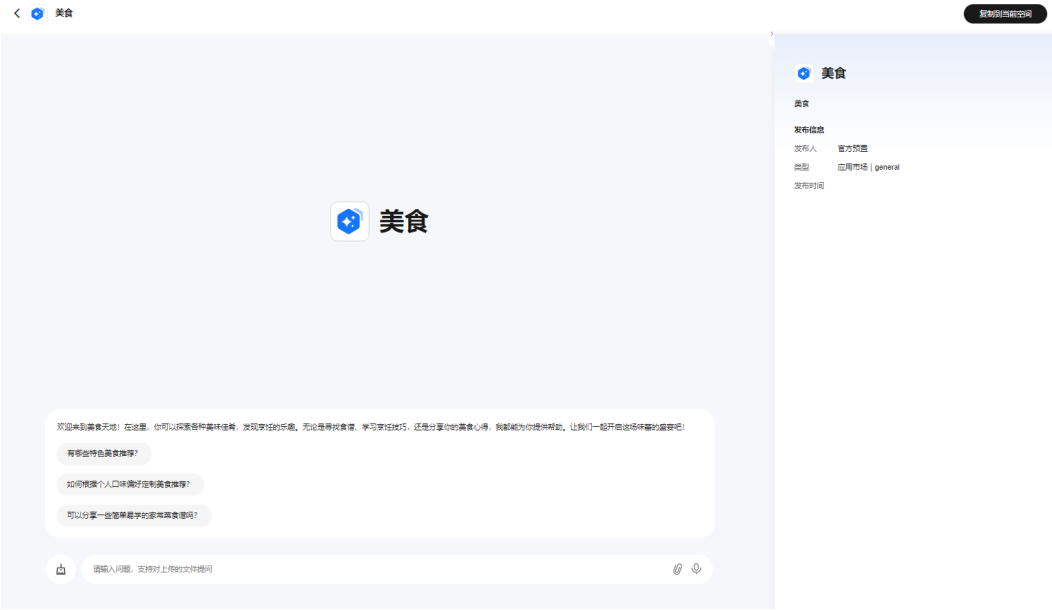
图 3-2 美食智能体
