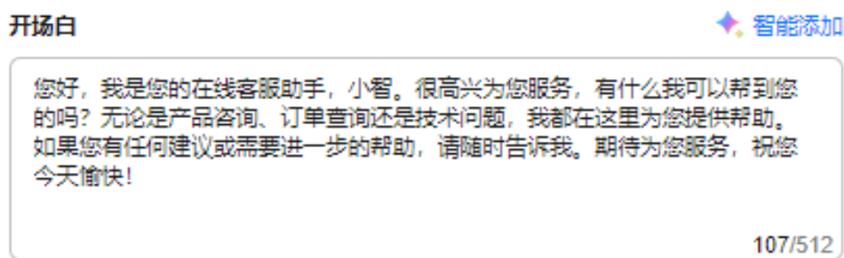
图 1-9 添加开场白
