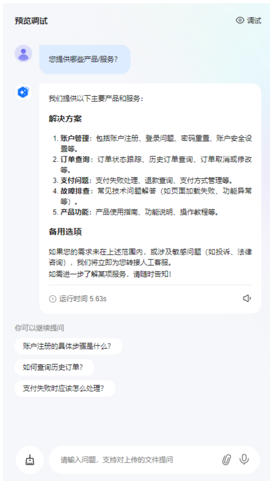
图 1-10 调试智能体
