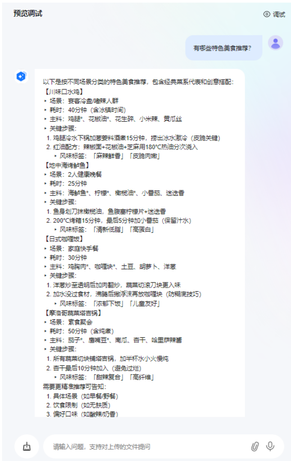
图 3-4 调试智能体
